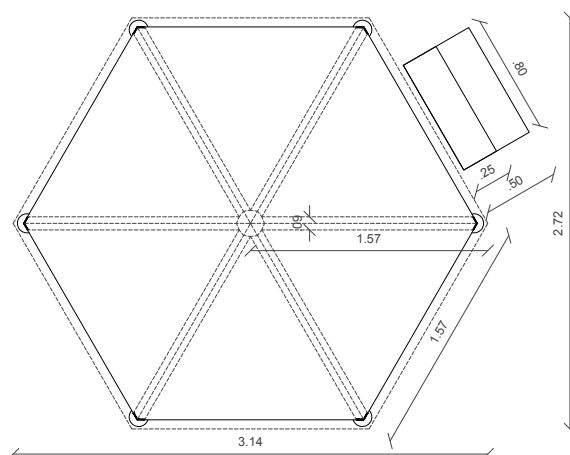
Corte e Planta, escala 1:50
